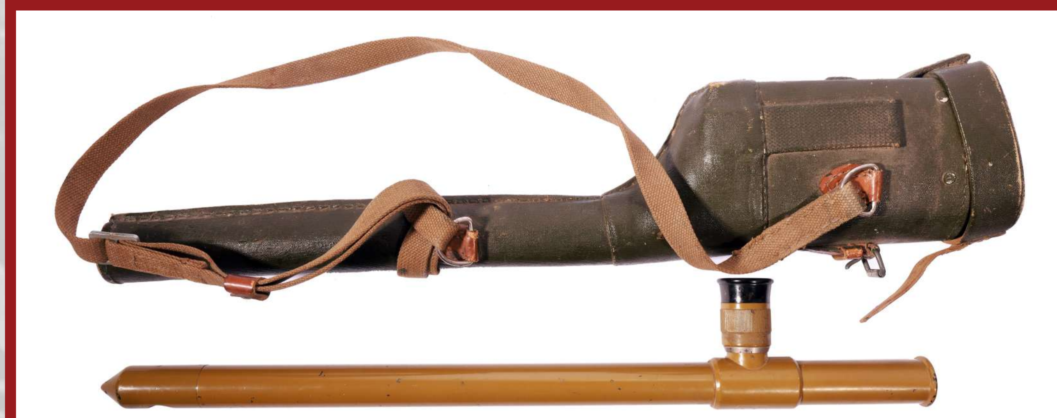
Перископ разведчика окопный оптический (с чехлом). РСФСР, 1941 г. Принадлежал генерал-полковнику В. Д. Цветаеву.
