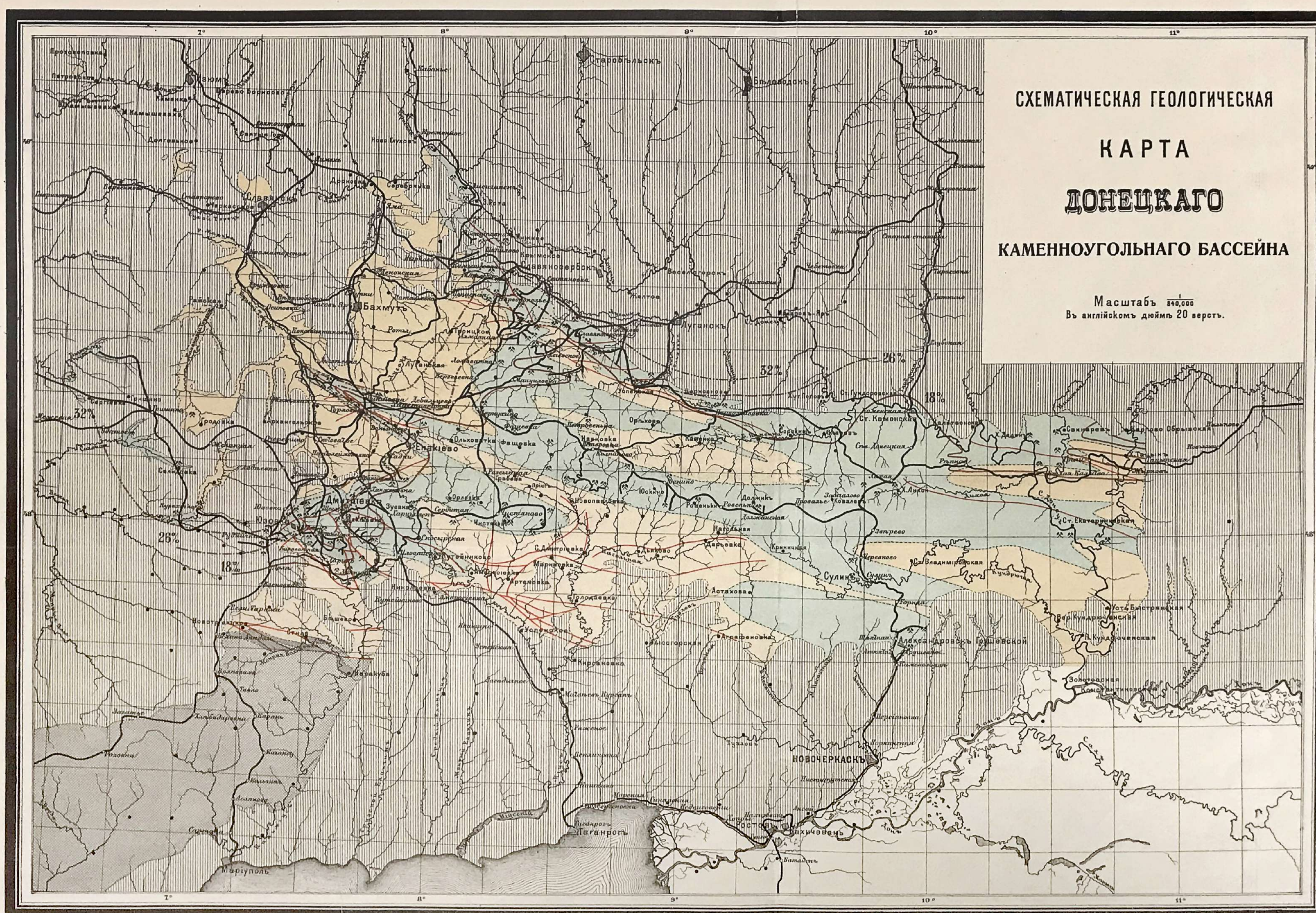
Схематическая геологическая карта Донецкого каменноугольного бассейна. Российская империя, не позднее 1917 г.
